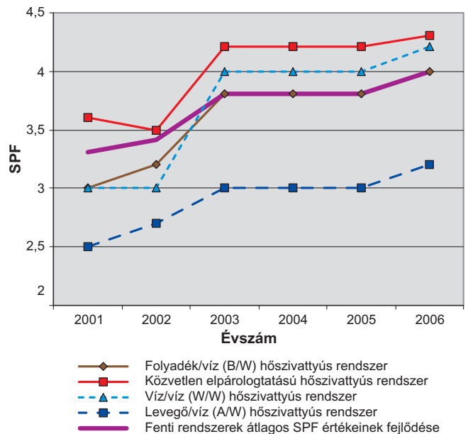
2. ábra. Különböző hűszivattyú típusoknál a teljes rendszerek szezonális teljesítmény-tényezőinek (SPF) fejlődése 2001 és 2006 között
