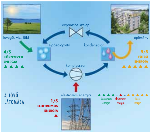
1. ábra. Hűszivattyús rendszerű energiahatékonyságnövelés
